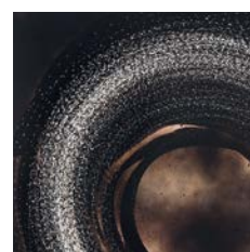
Milky Way » 26
